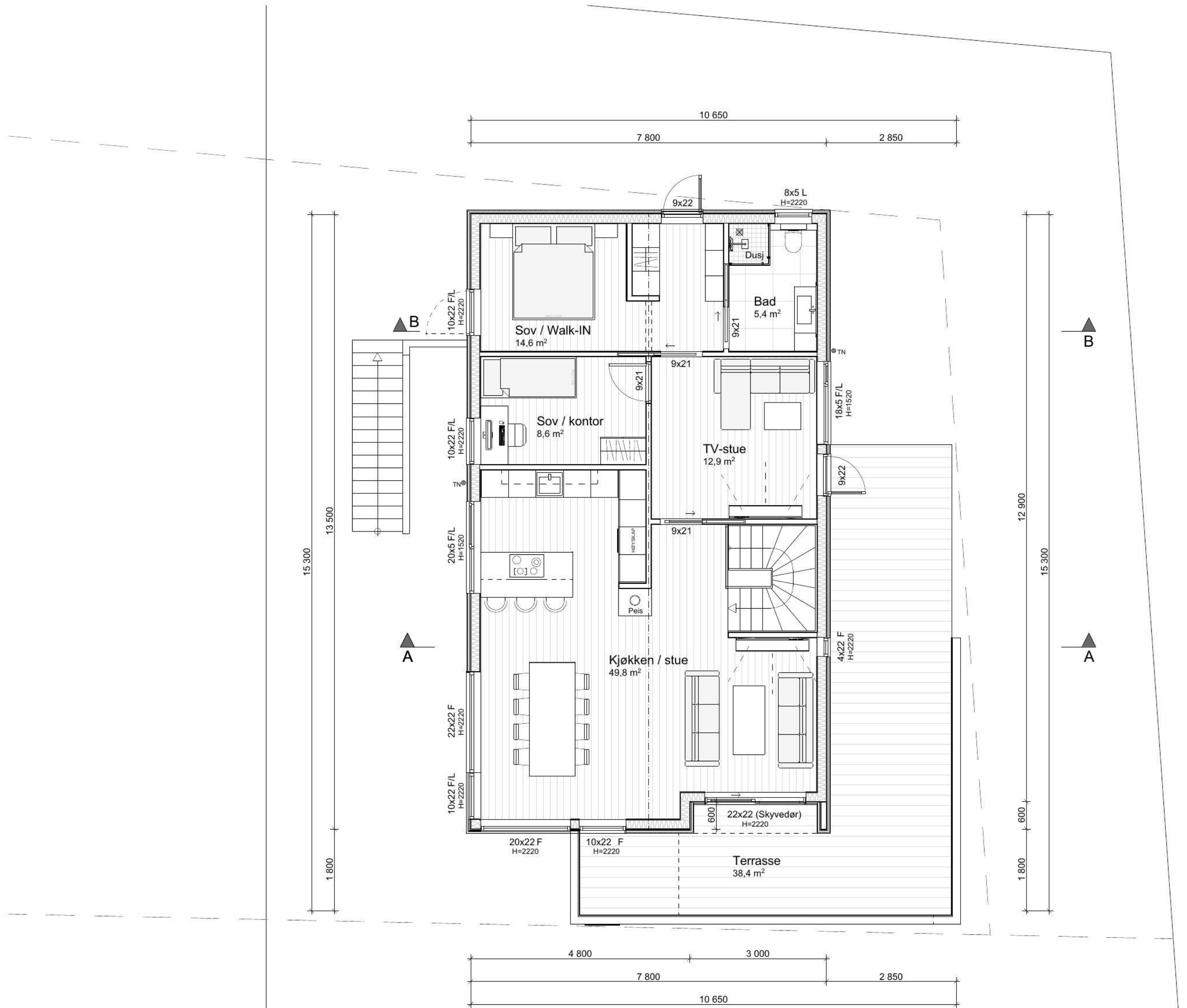
Plan 2.etasje BRA bolig A 94,6 m²
